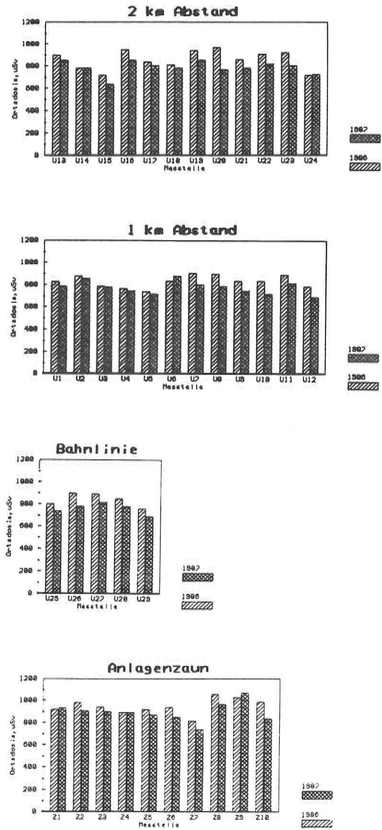
Abb. 4 Jahres-Ortsdosis in der Umgebung der Schachtanlage Asse 1986 und 1987 (in \mu\text{Sv} )
